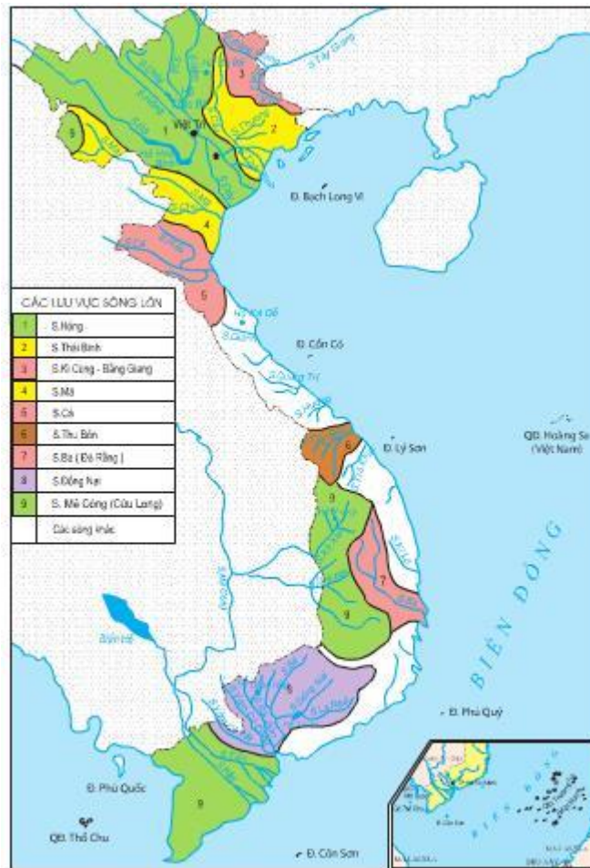
Hình 33.1. Lược đồ các hệ thống sông lớn ở Việt Nam
