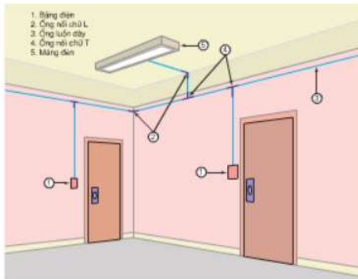
Hình 11 - 1. Mạng điện tập thể kiểu mở trong ống cách điện.
