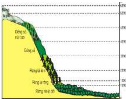
đet - Hình 46.2 - Sơ đồ sườn đông An-đét qua lãnh thổ Pê-ru
