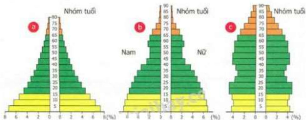
Hình 48. Ba dạng tháp tuổi (%)
